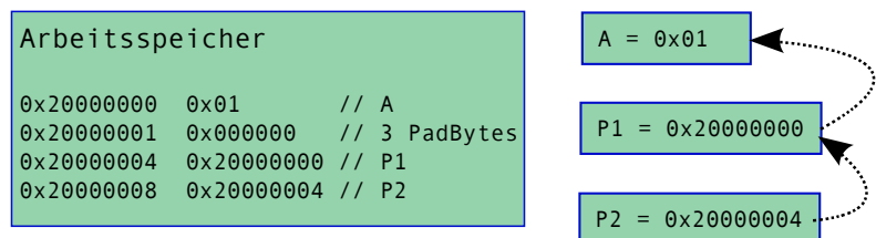
Zeiger auf Abbildung 3: Zeiger in C
